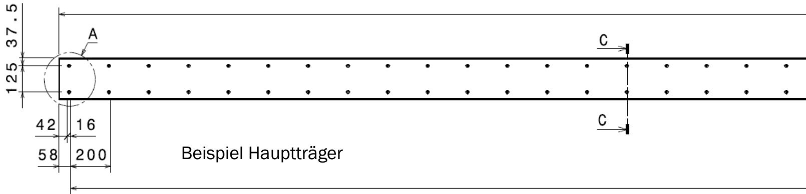
Beispiel Hauptträger
