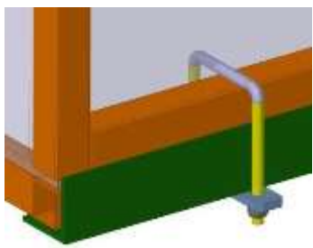
Befestigung mit Standard U-Bügel
