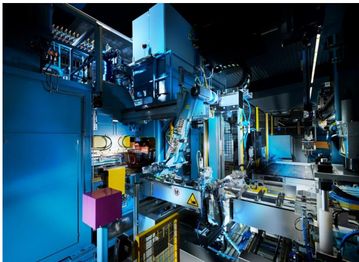
Abb. 2: Über diese Zuführung erfolgt der Transport der drei aufeinandergelegten Bleche in die Buckelpresse, die für deren Verbindung eine hohe Zahl von Schweißbuckeln hochpräzise verschweißt. Foto: NIMAK GmbH
