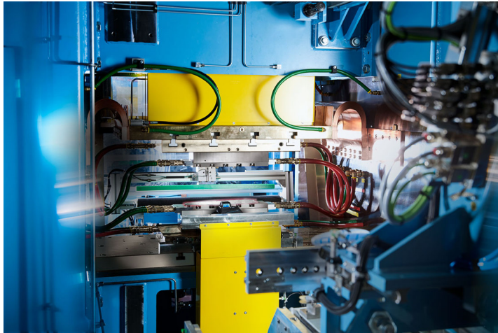
Abb. 3: Die Buckelpresse der NIMAK-Portalanlage verfügt über eine extrem hohe Elektrodenkraft und ist mit einem hydraulischen Antrieb ausgestattet. Dieser ist regelbar und ermöglicht so die Einstellung von Kraftprofilen. Foto: NIMAK GmbH
