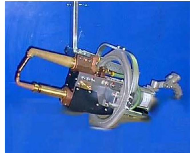
Kabel-Handzangen
