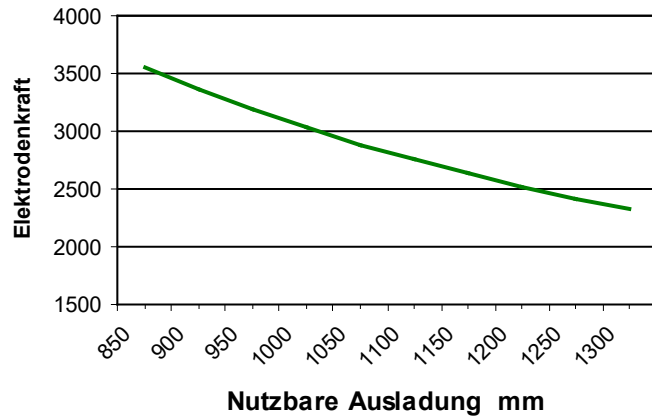
max.Elektrodenkräfte bei 4bar
