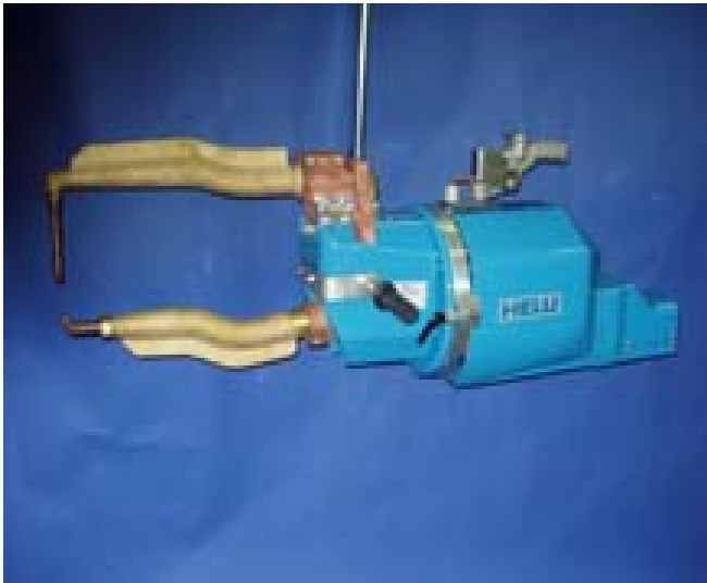
Integrierter Transformator
