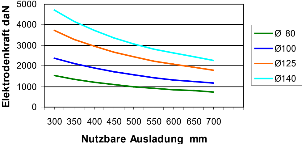
Elektrodenkräfte bei 5 bar
